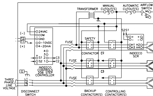
Finned Tubular
